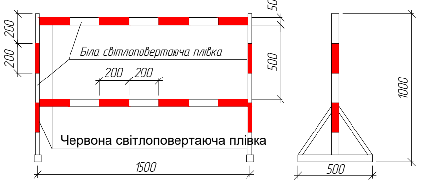
Огороджувальний бар'єр
