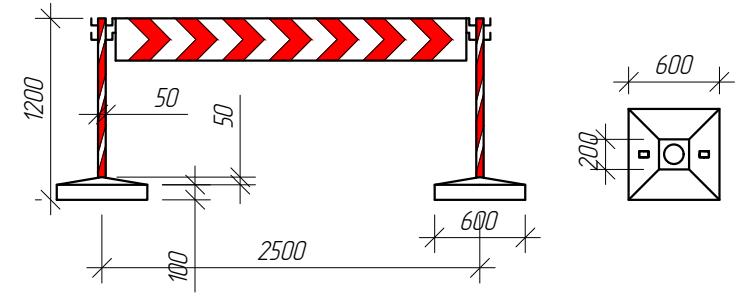
Поперечний бар'єр
