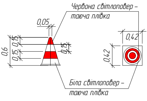
Напрямний конус
